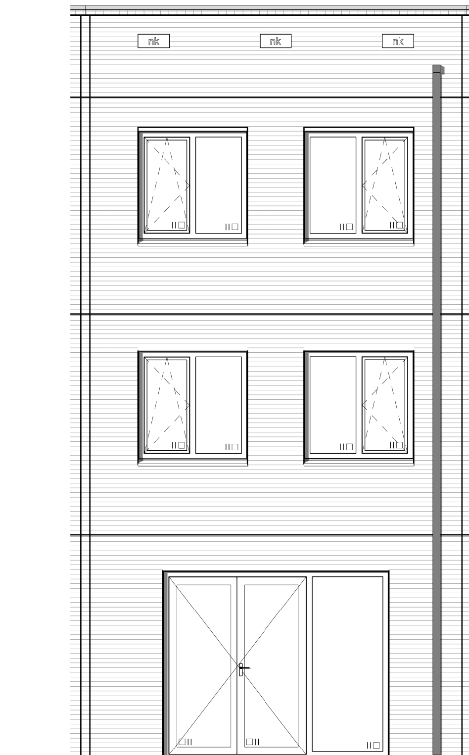
achtergevel
