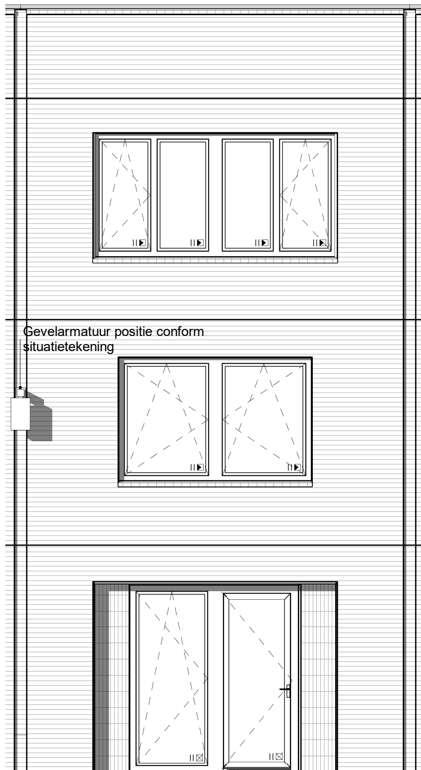
voorgevel
