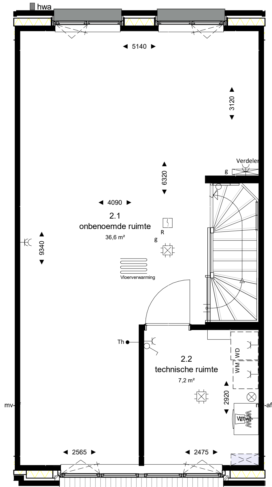
tweede verdieping
