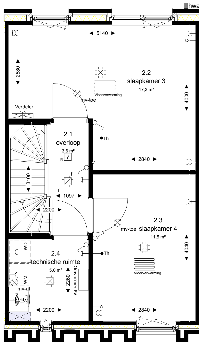
tweede verdieping
