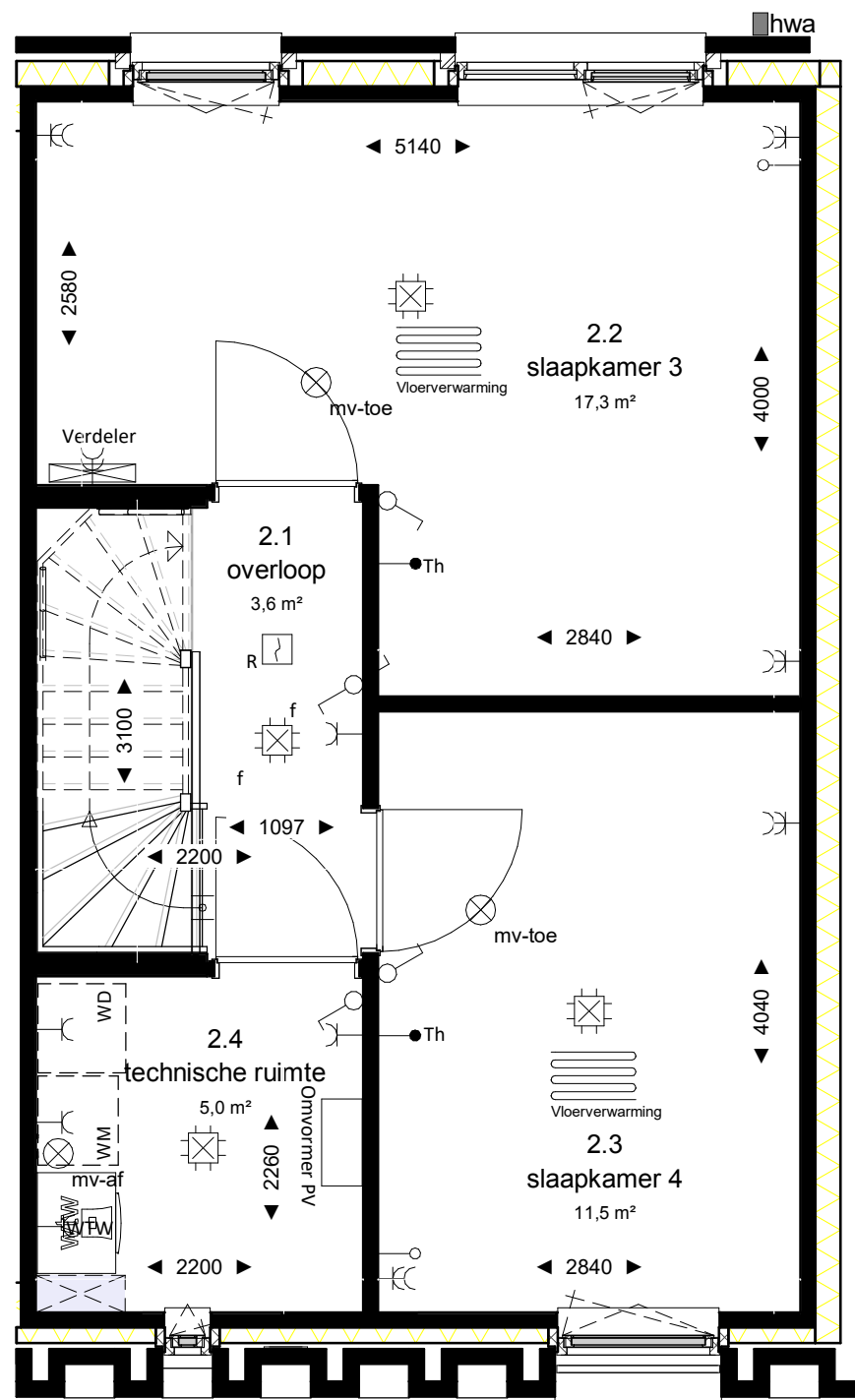
tweede verdieping
