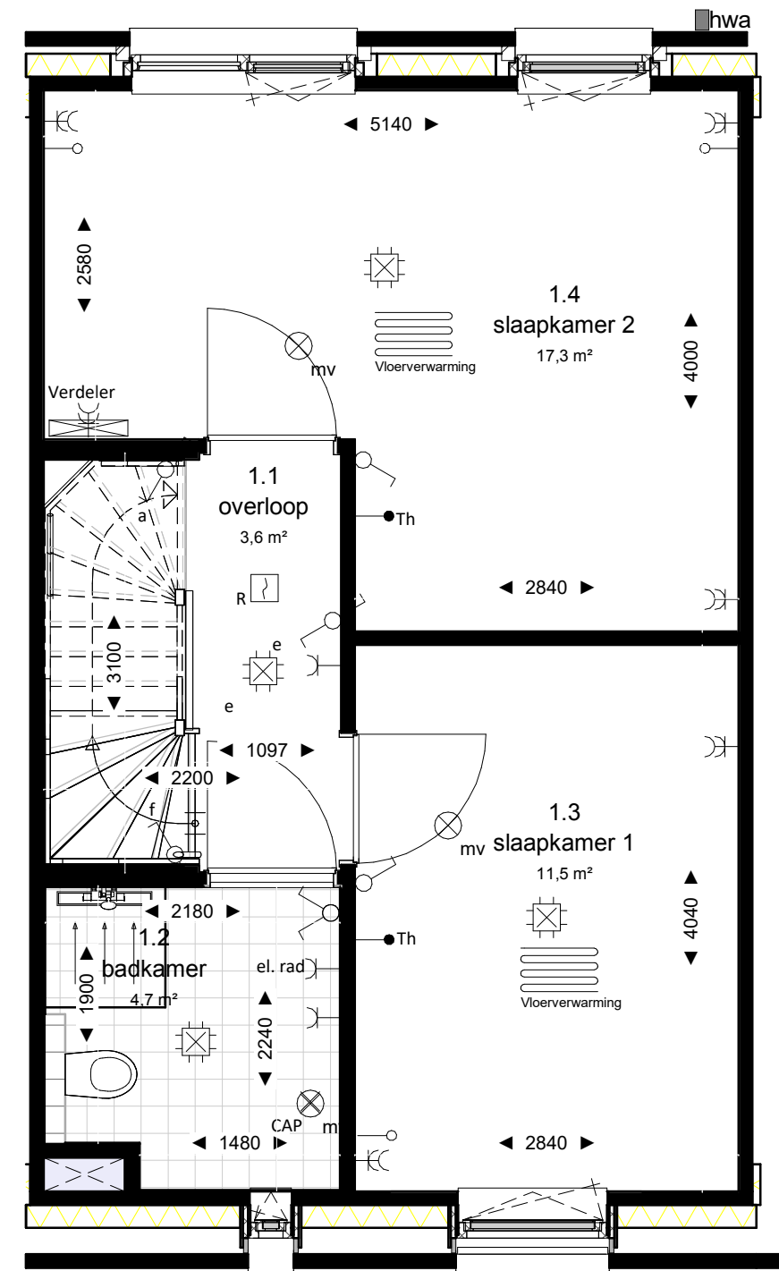
eerste verdieping
