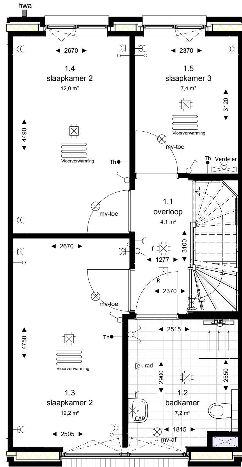
eerste verdieping
