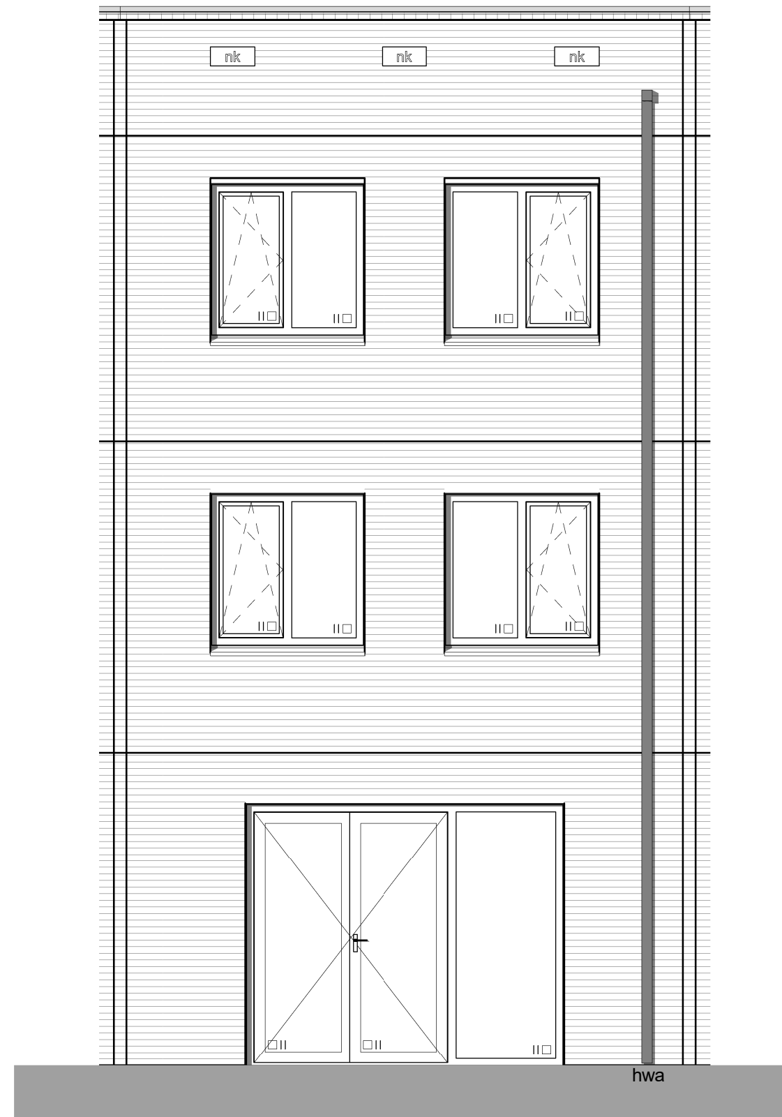
achtergevel
