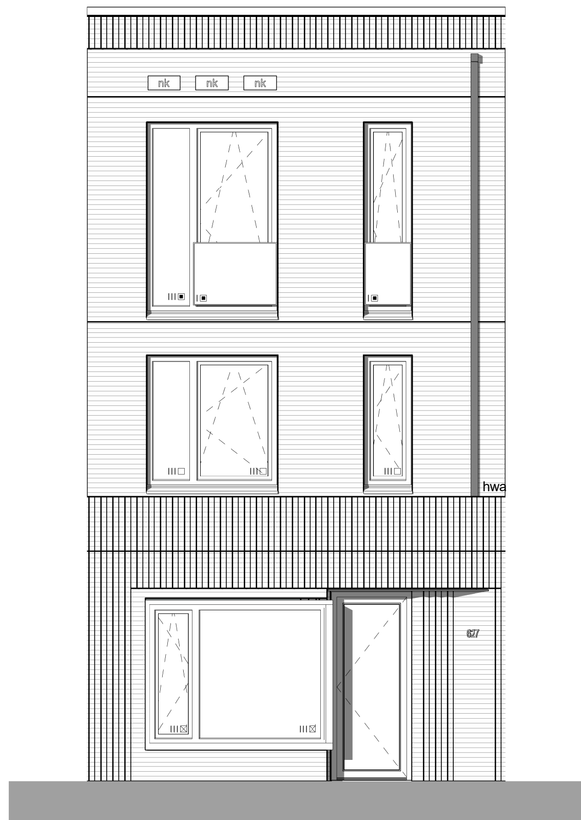
voorgevel
