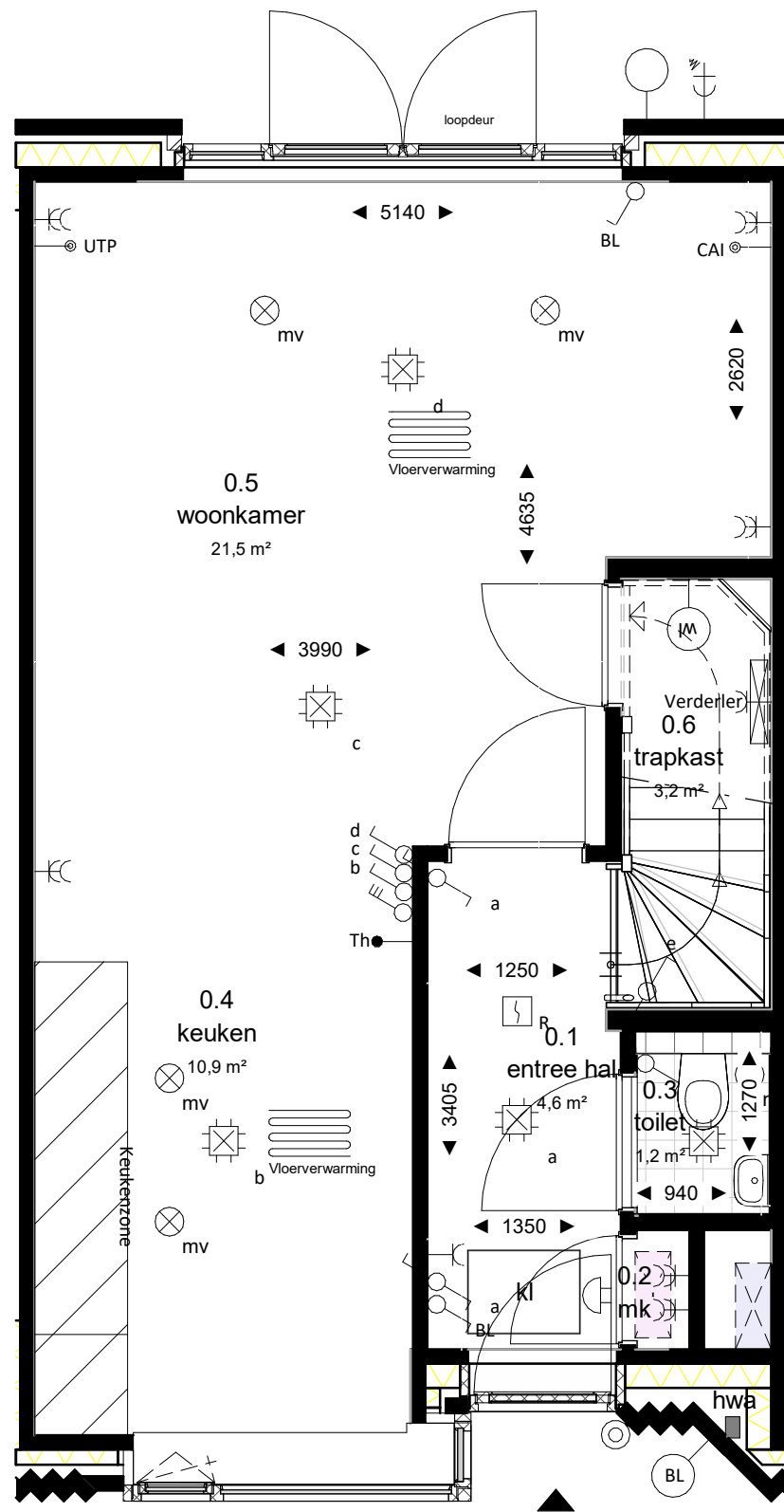
begane grond
