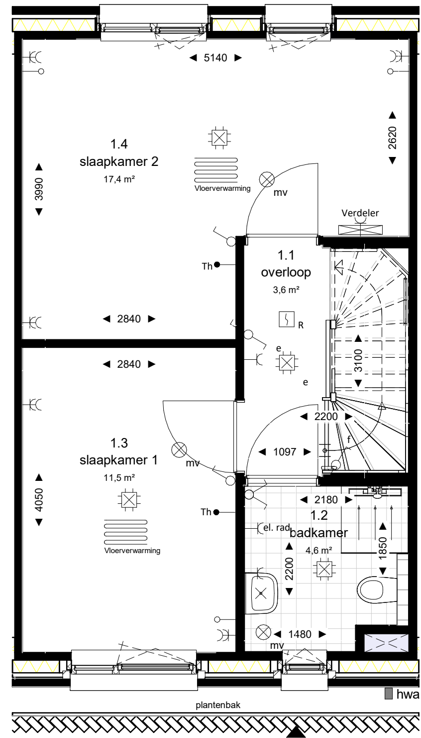
eerste verdieping
