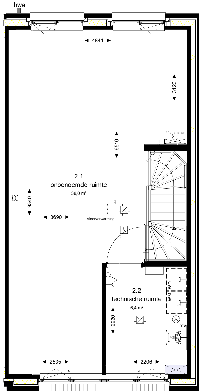
tweede verdieping
