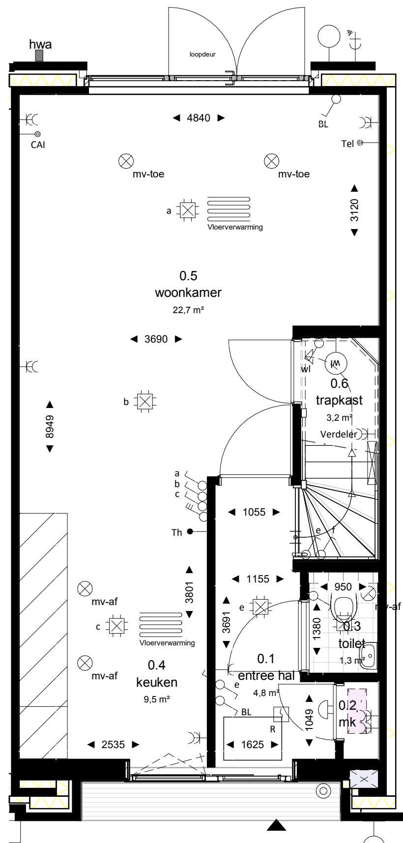
begane grond
