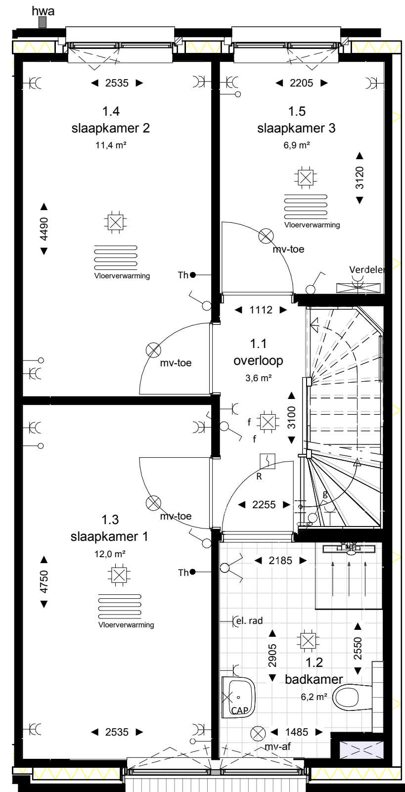
eerste verdieping
