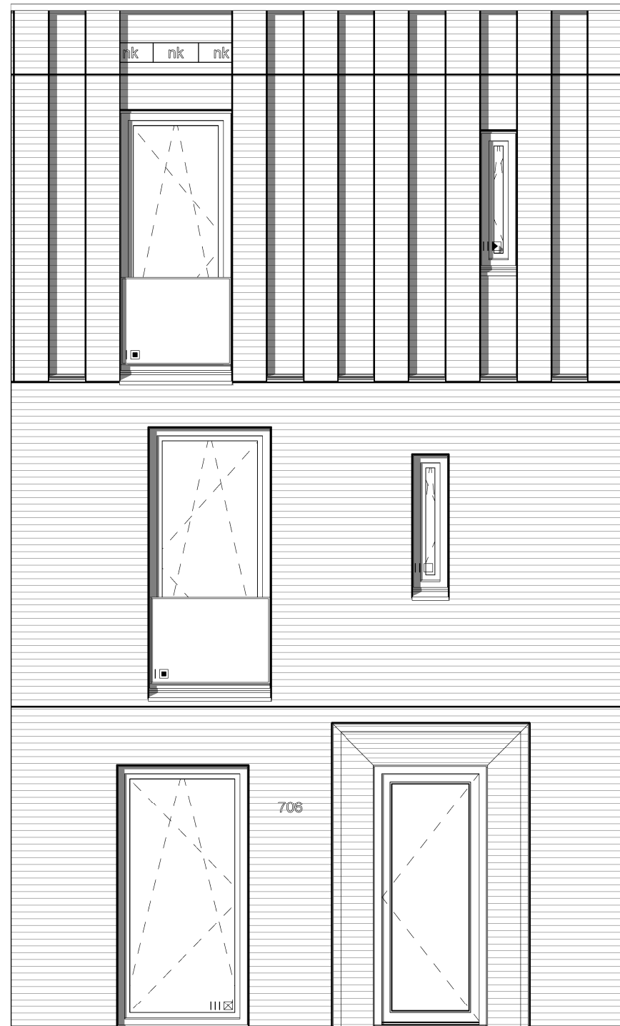
voorgevel
