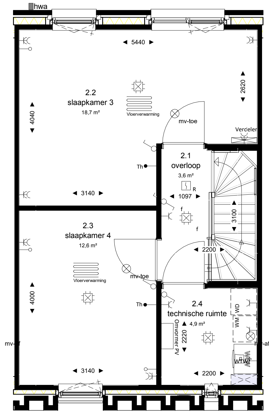
tweede verdieping
