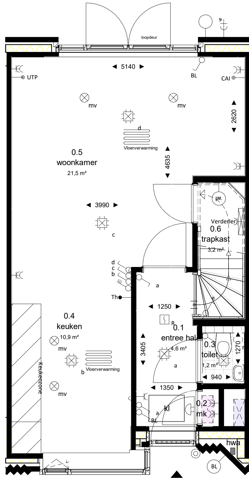
begane grond
