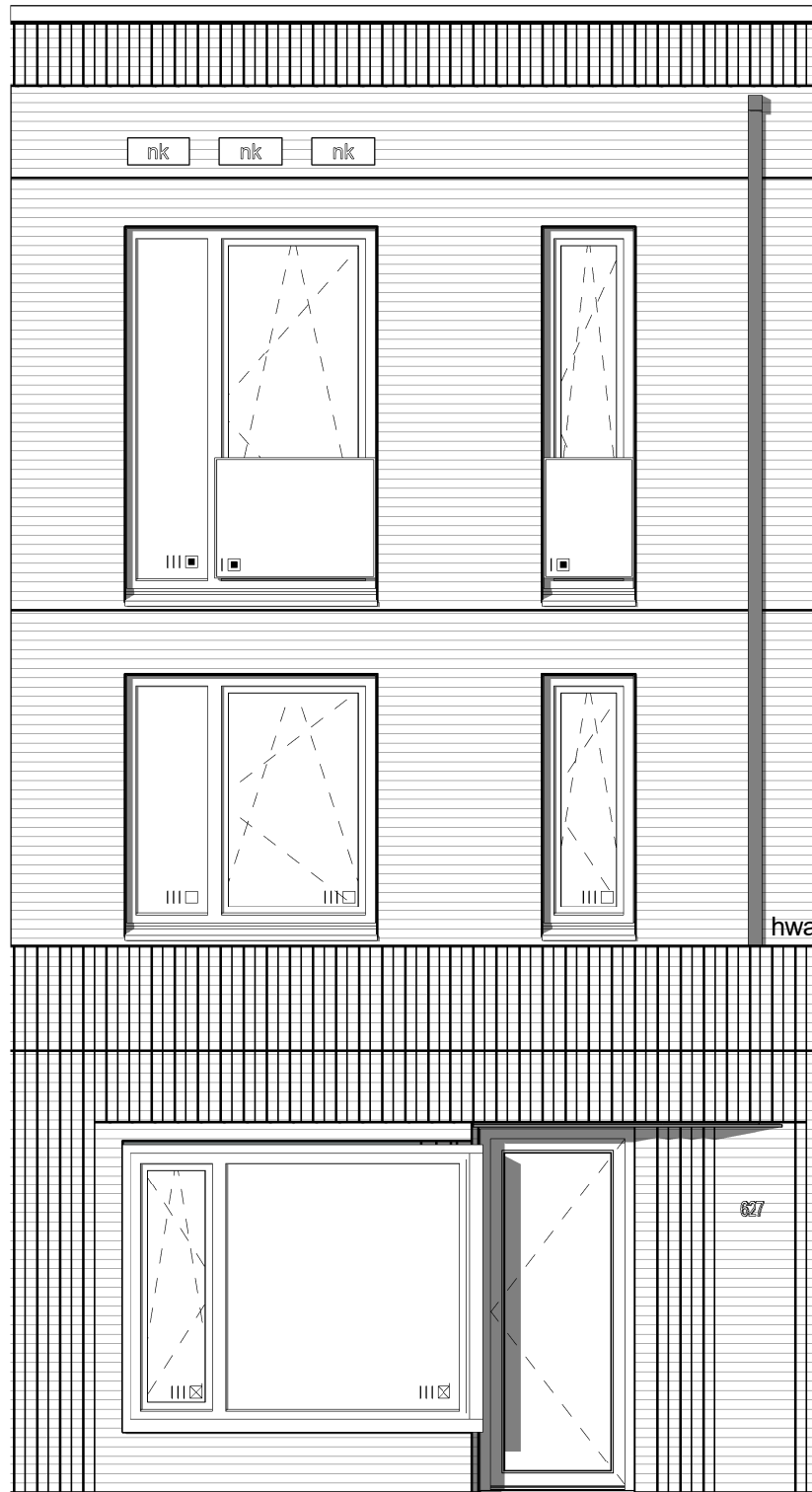
voorgevel
