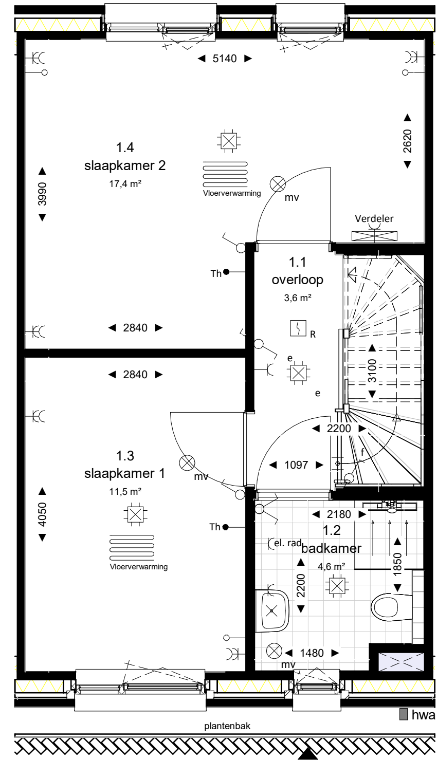
eerste verdieping
