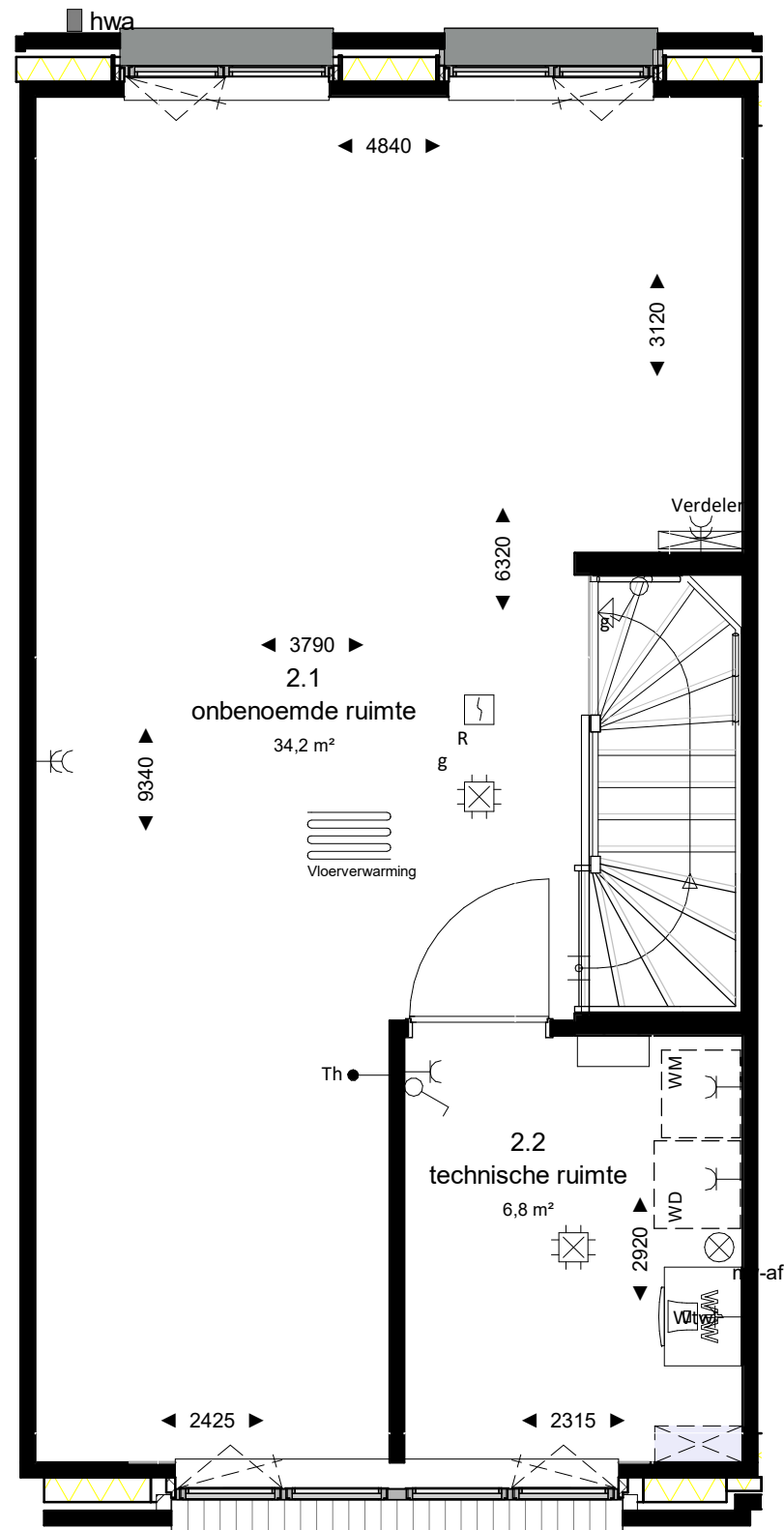
tweede verdieping
