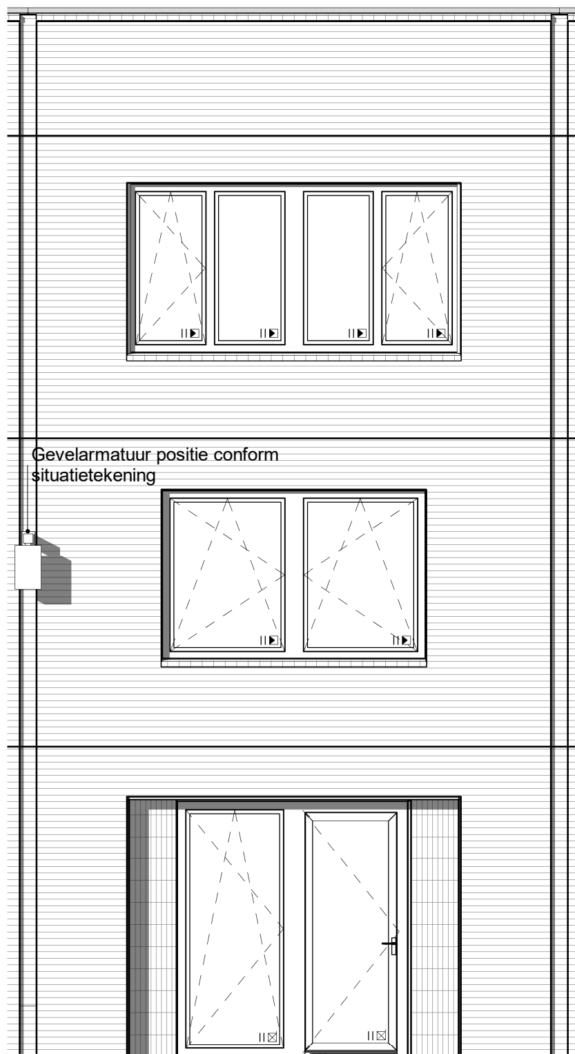
voorgevel
