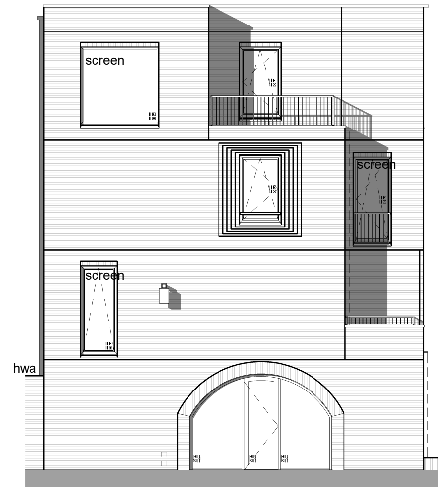
linkergevel
