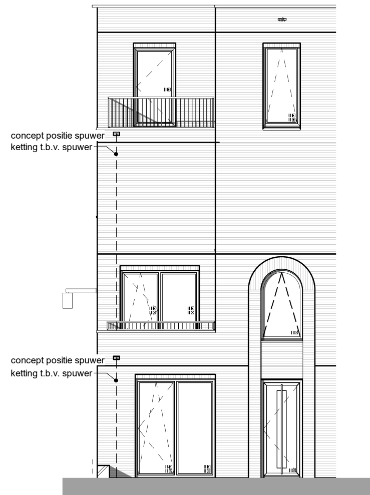
voorgevel
