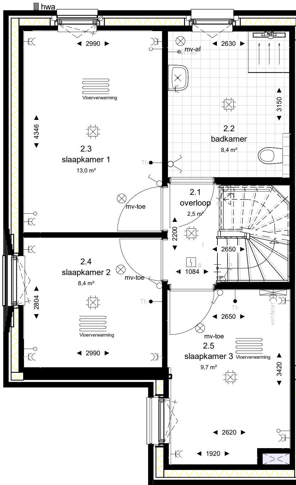
tweede verdieping
