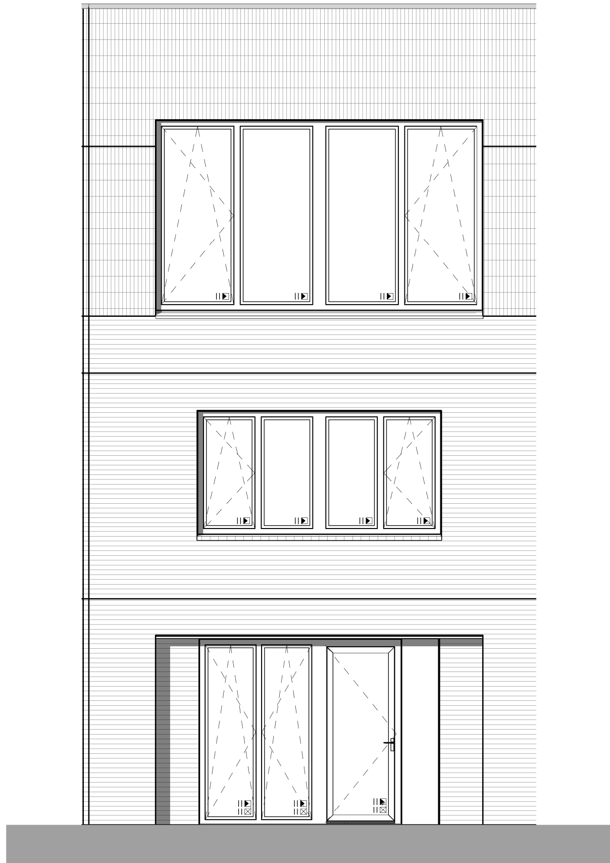
voorgevel
