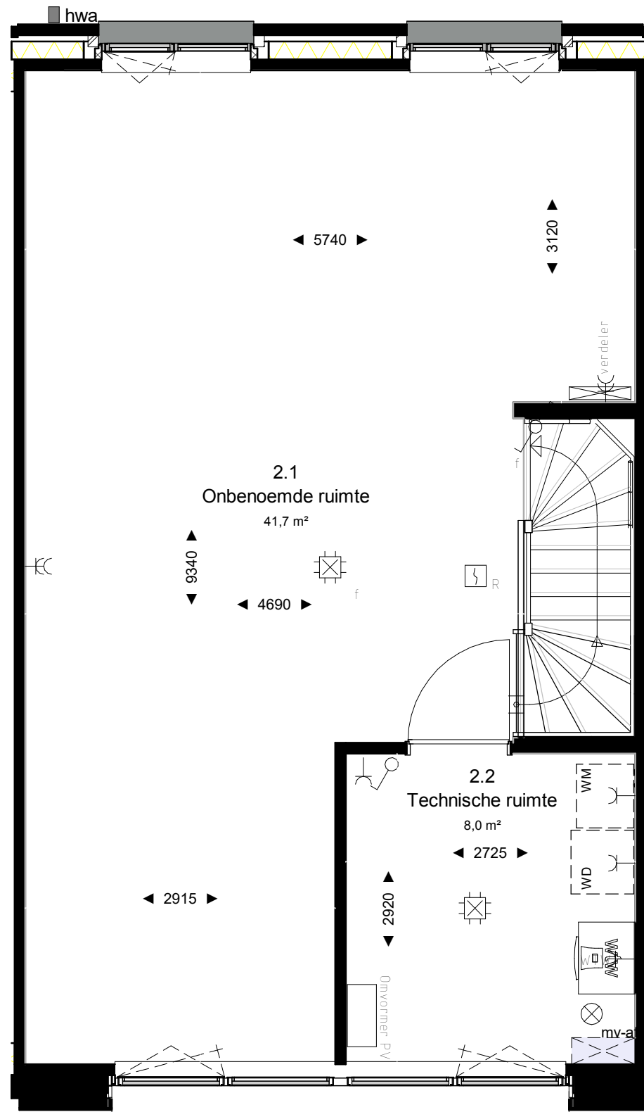
tweede verdieping
