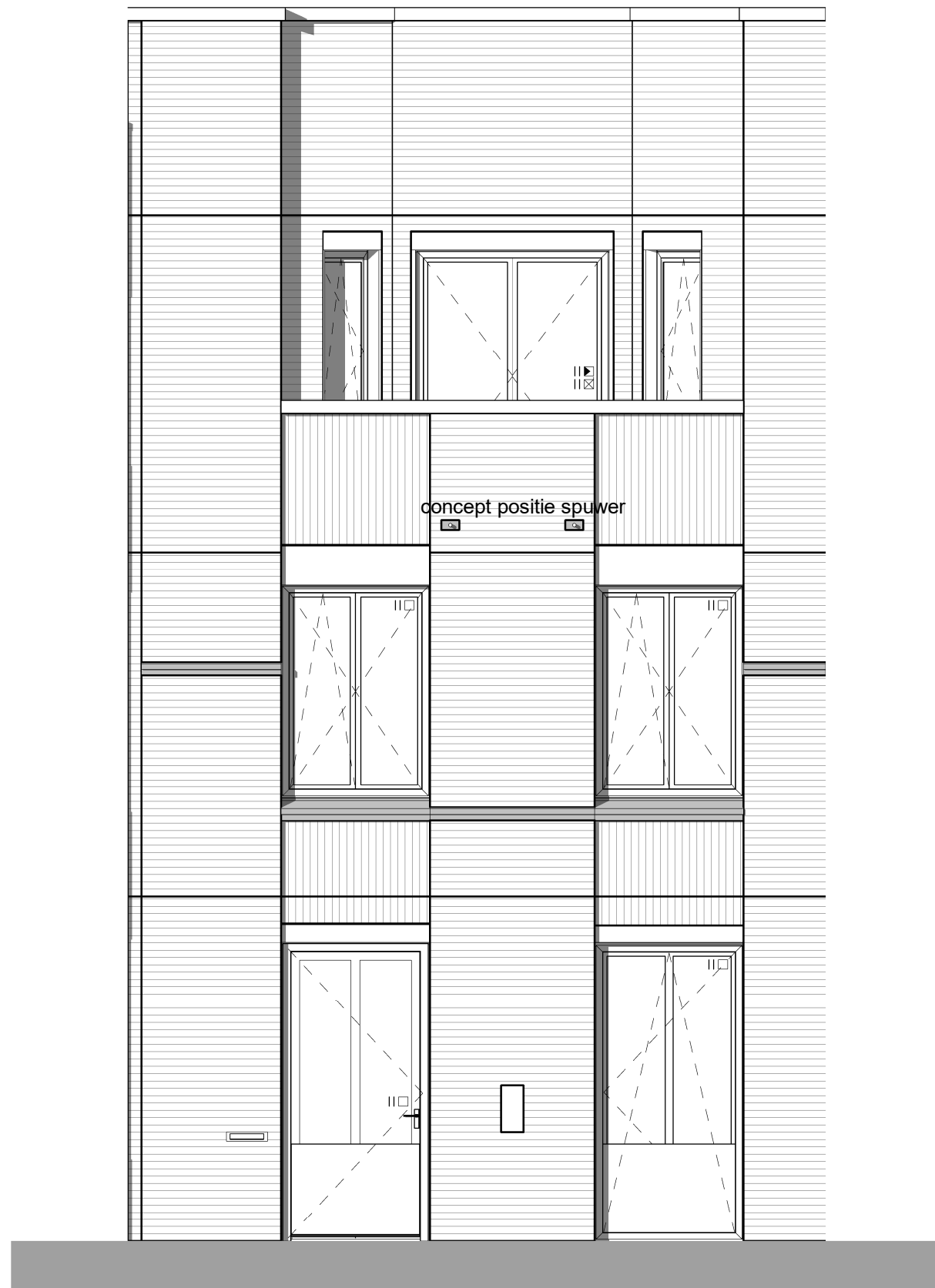
voorgevel
