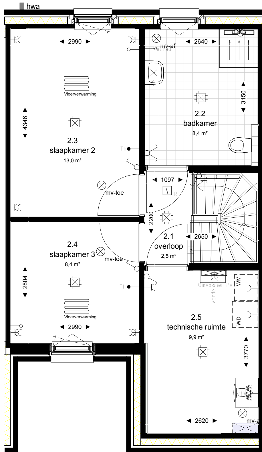
tweede verdieping
