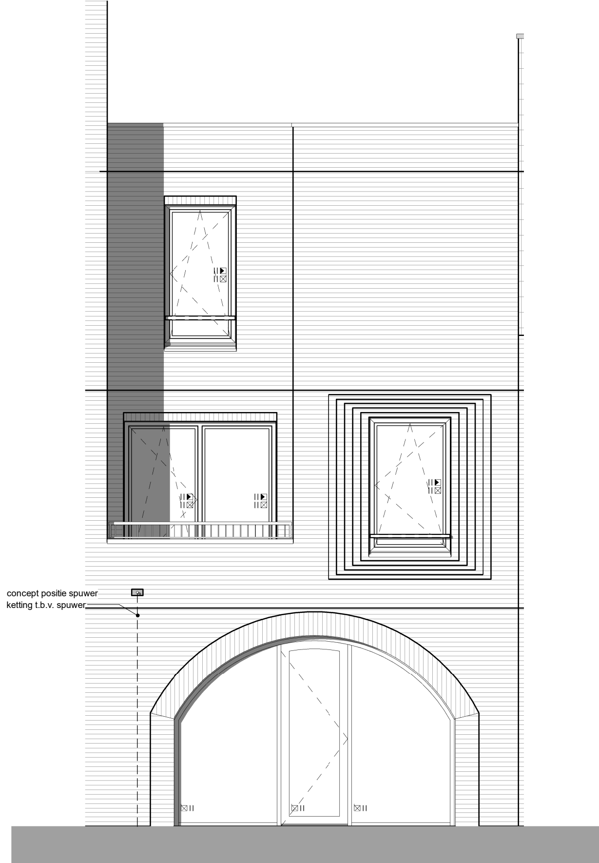
voorgevel
