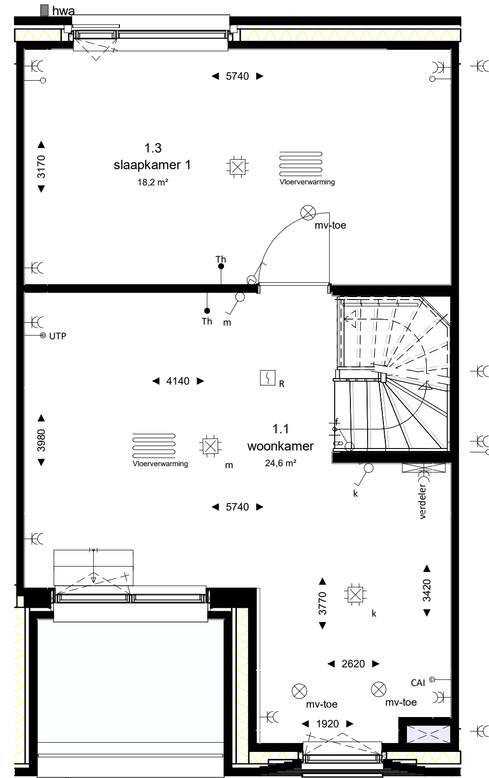
eerste verdieping
