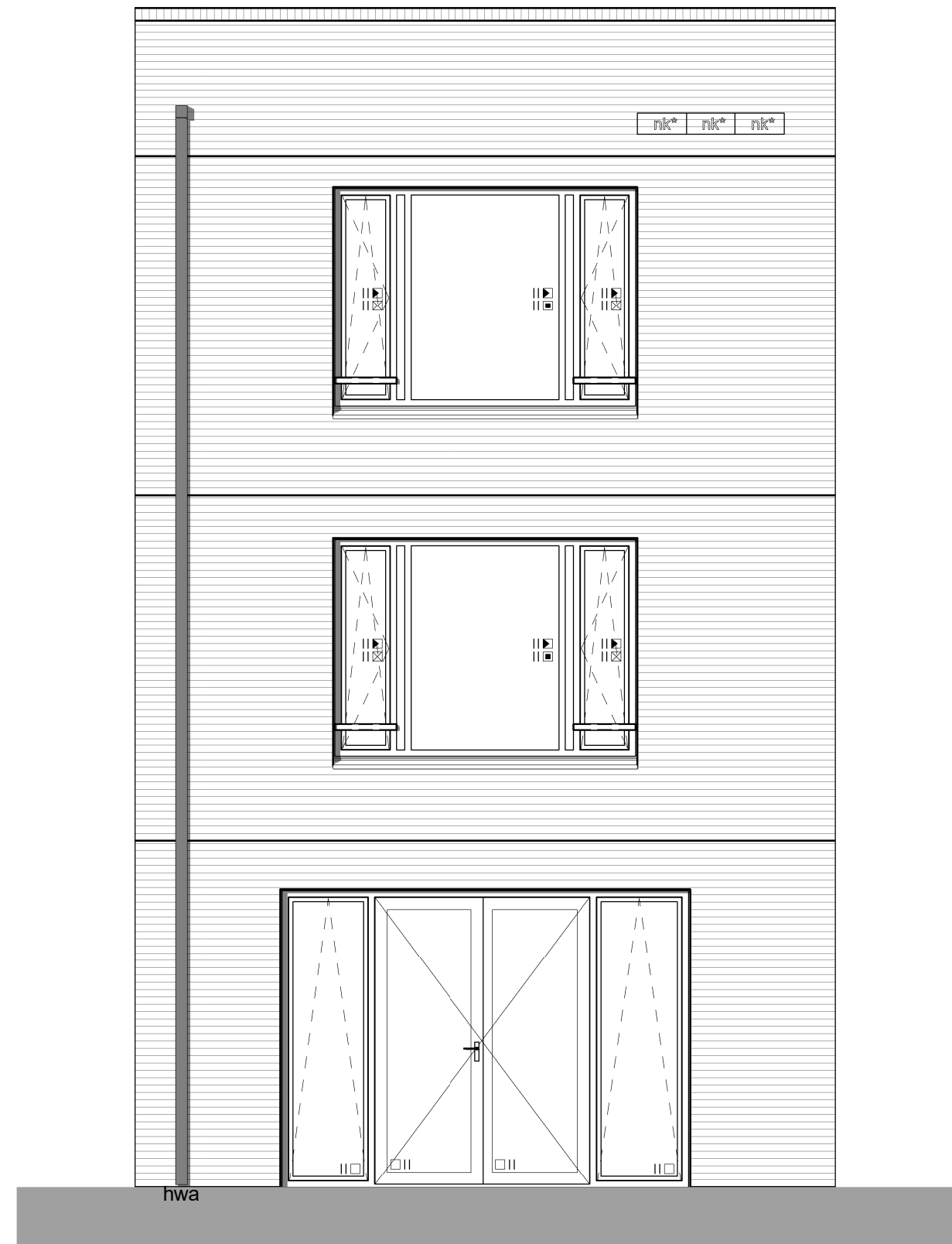
achtergevel
