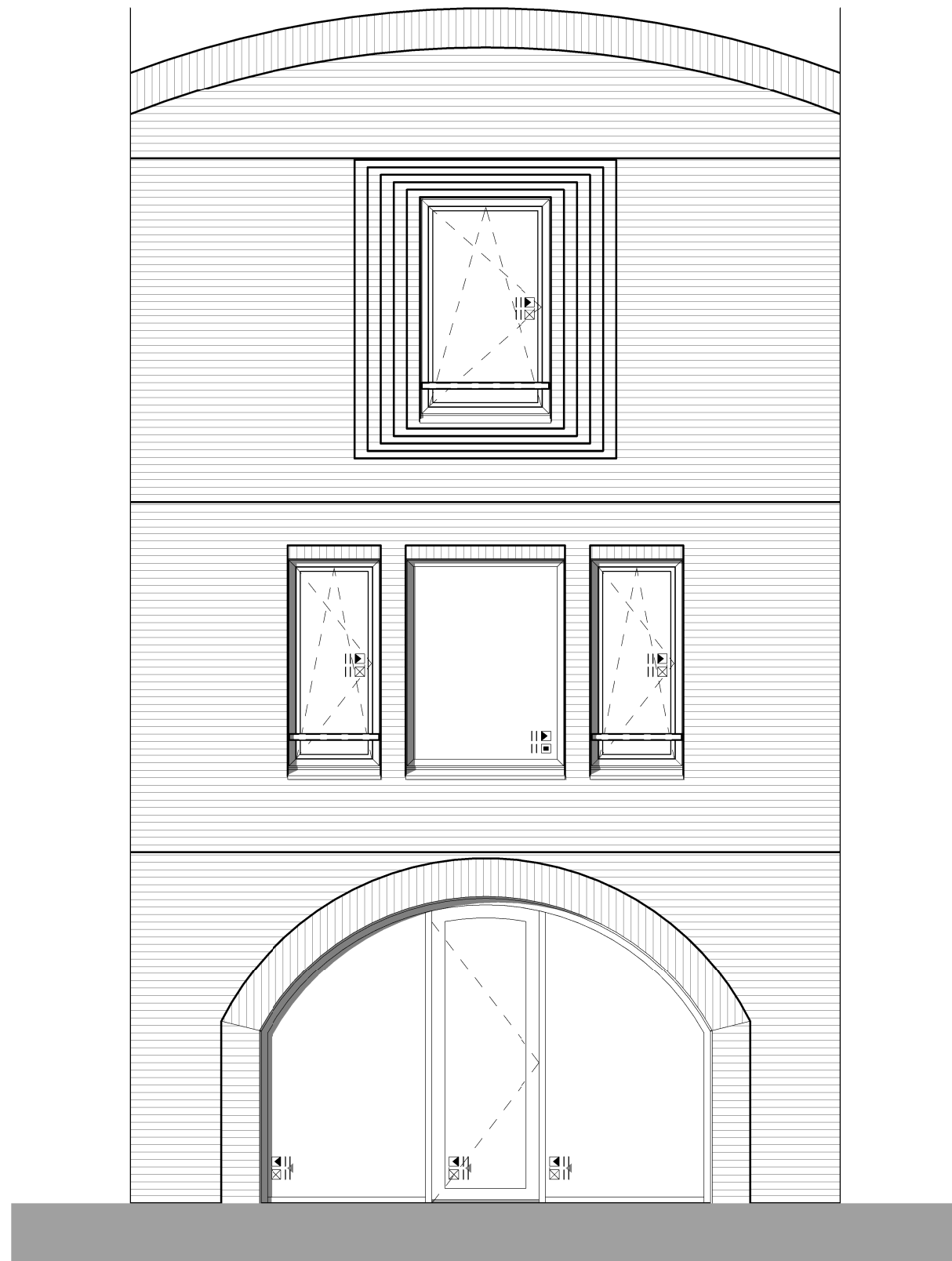
voorgevel
